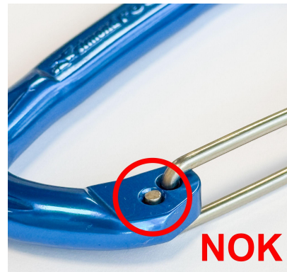
Rivetage NOK, extrémité plate
